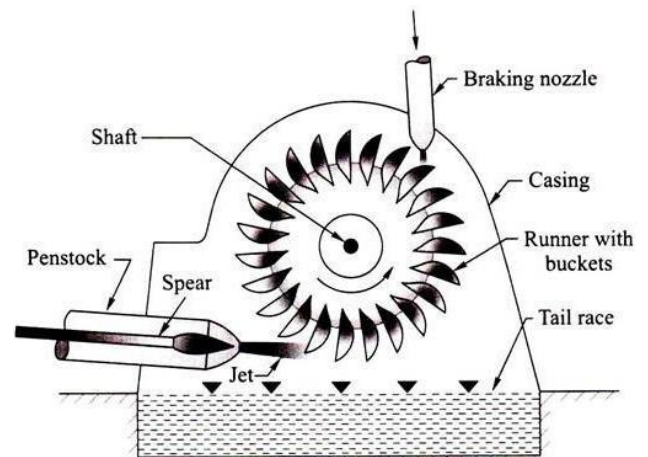
Fig. 24. Pelton turbine
