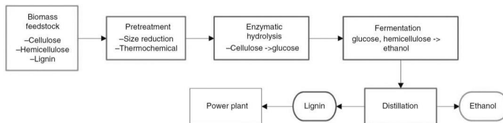
Fig. 9. Ethanol Fermentation
