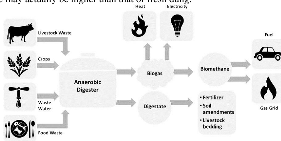
Fig. 7. Anaerobic Fermentation
