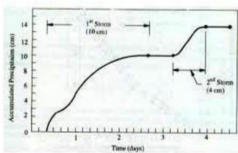
FIG:MassCurve ofRainfall
