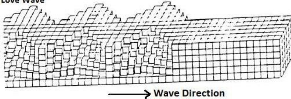
Love Wave
